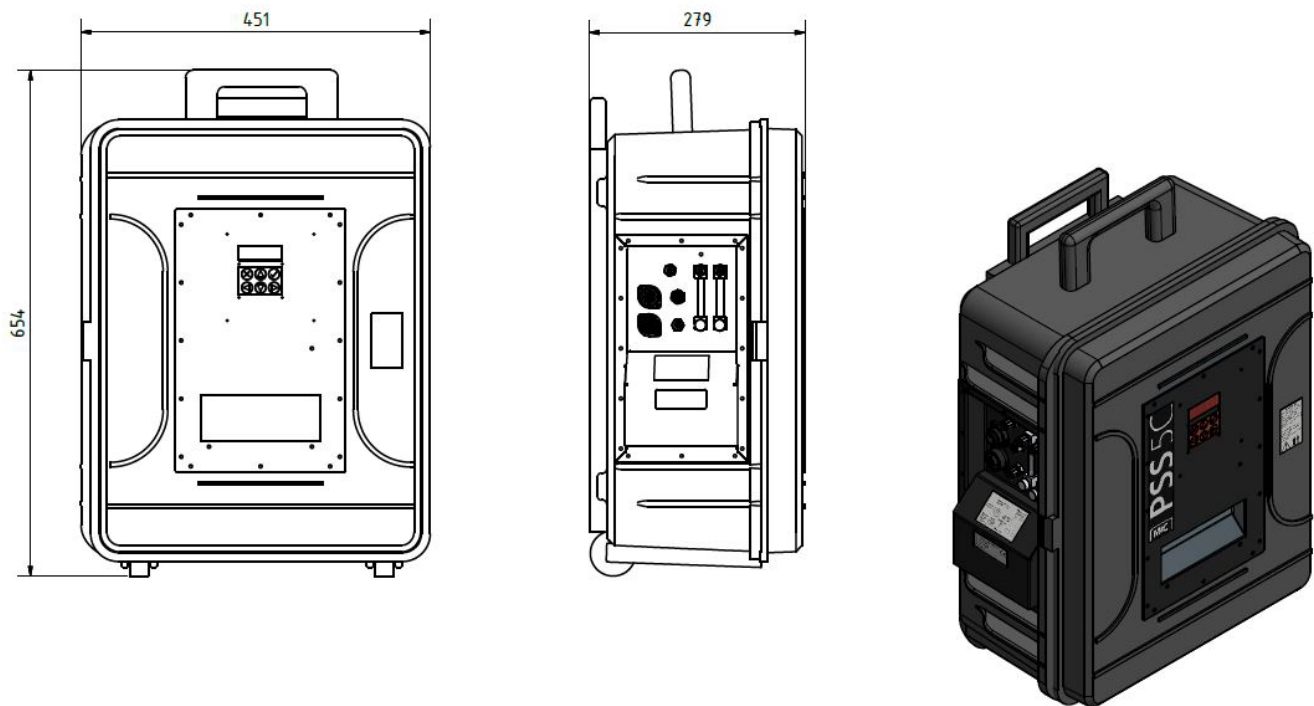
Abbildung 7 Abmessungen
