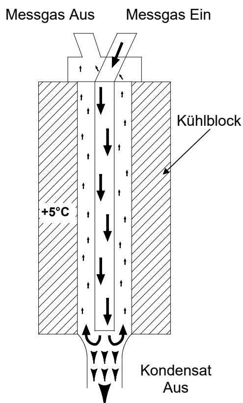
Abbildung 4 Funktion des M&C Jet-Stream-Wärmetauschers
